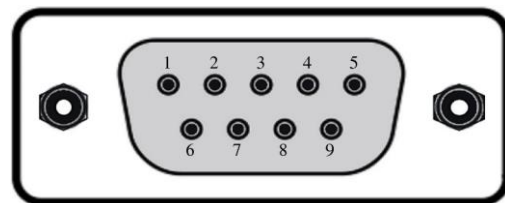
Steckerbelegung DSUB9 Stecker
